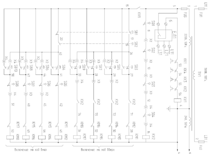
Рис. 3. Схема электрическая принципиальная подъемника ПП-16
